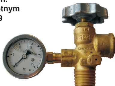
Zawór poboru fazy gazowej z manometrem REGO 9101
